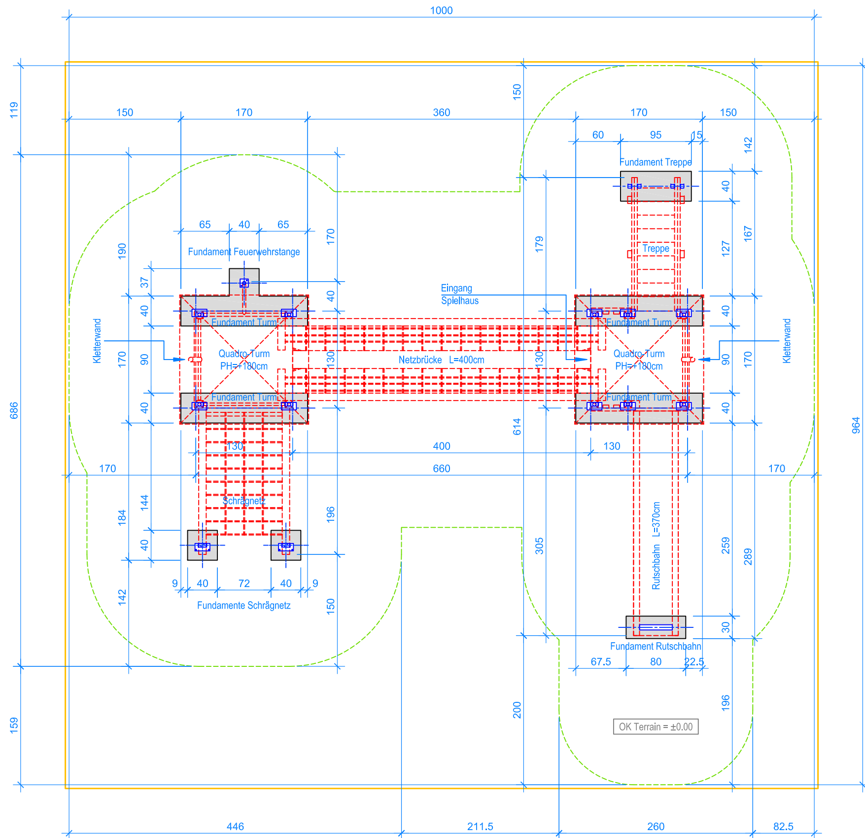
GRUNDRISS 1:50
