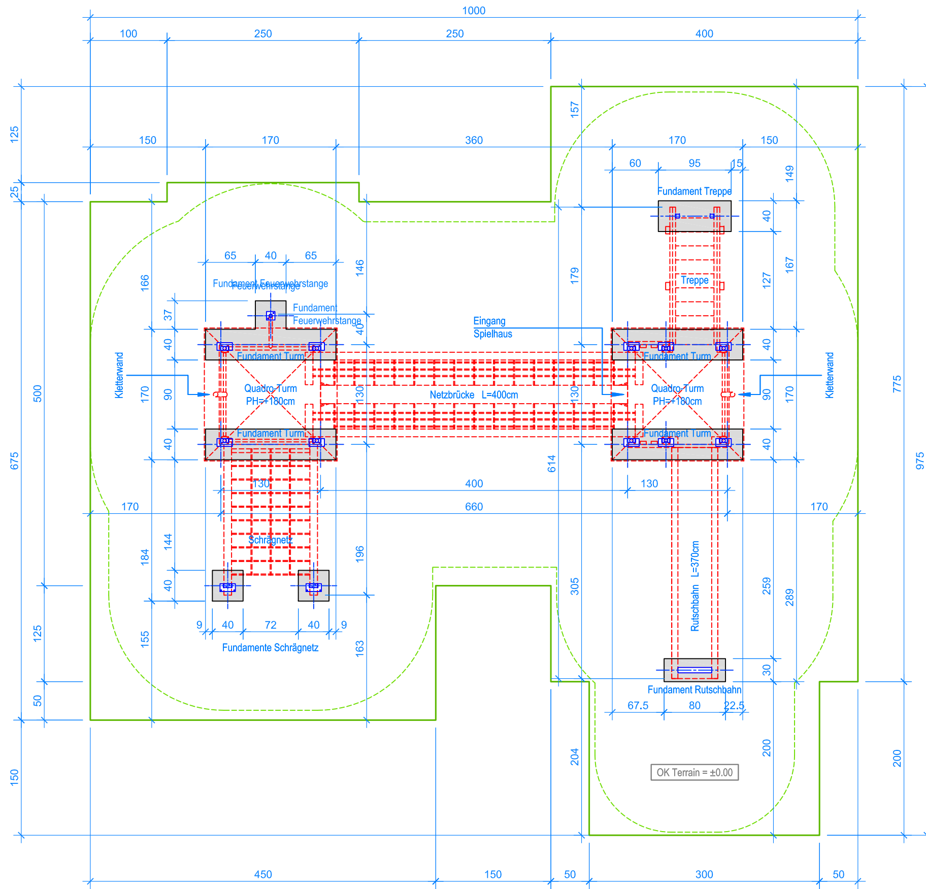
GRUNDRISS 1:50
