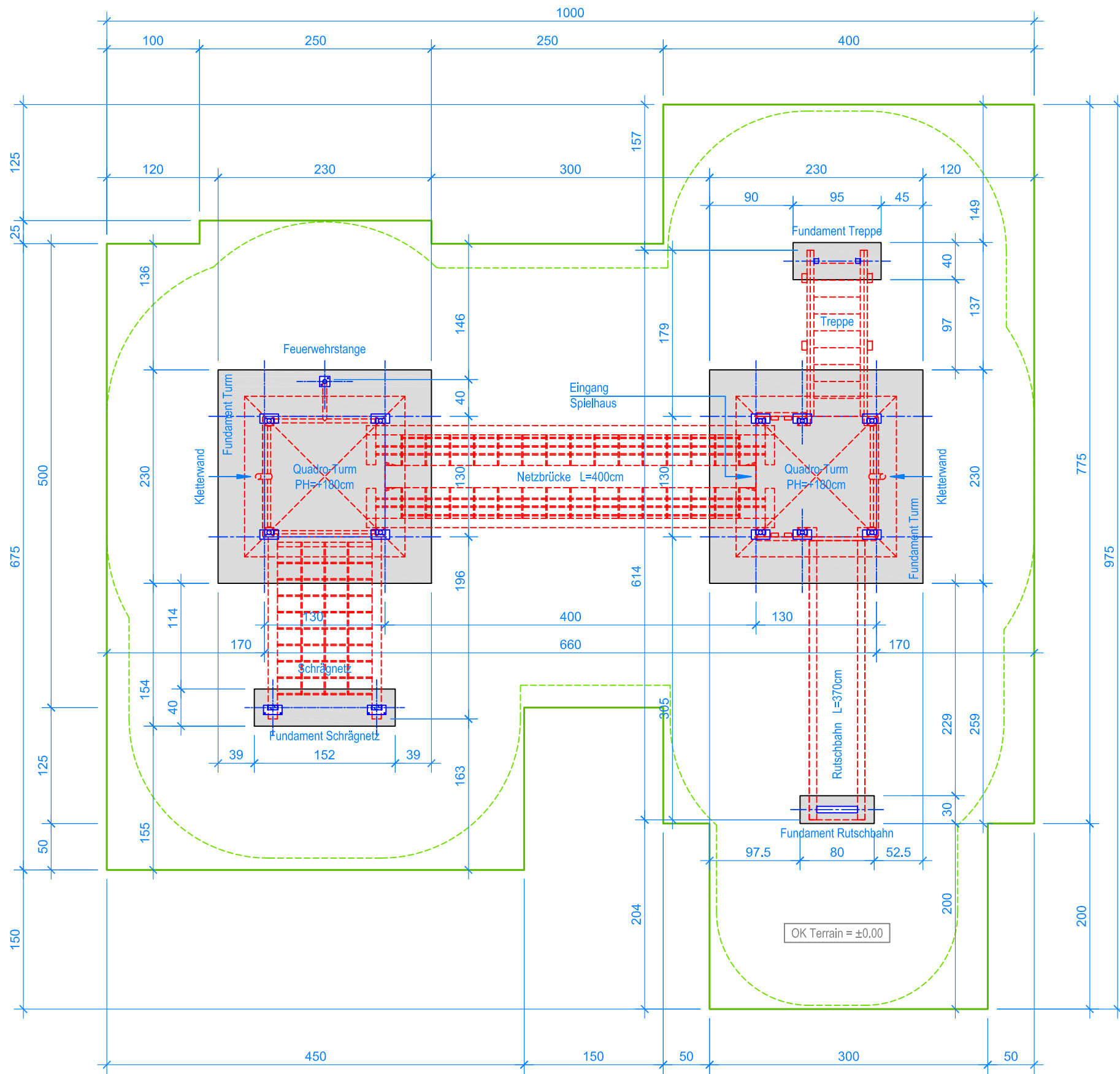
GRUNDRISS 1:50
