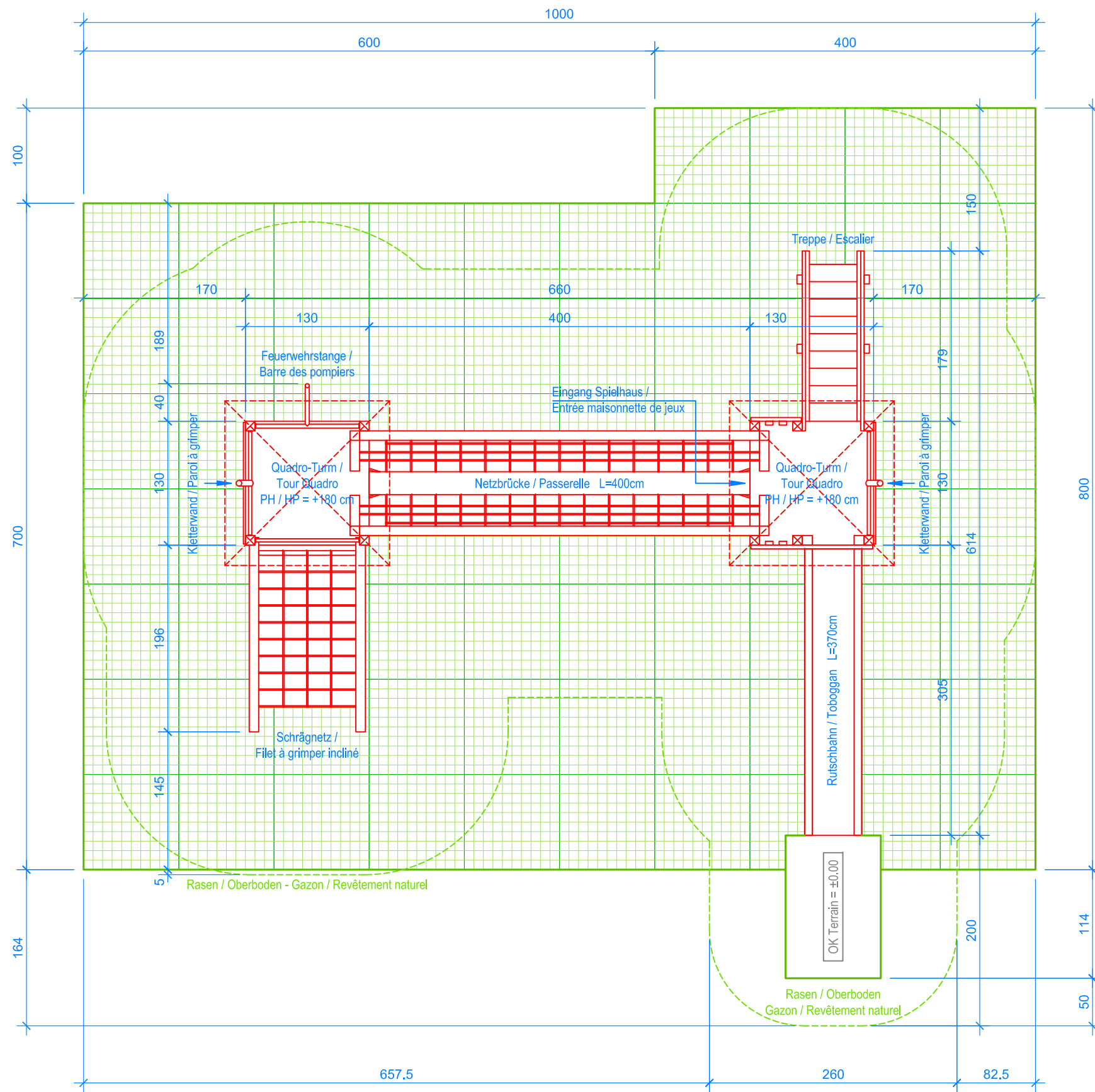
GRUNDRISS / PLAN 1:50
