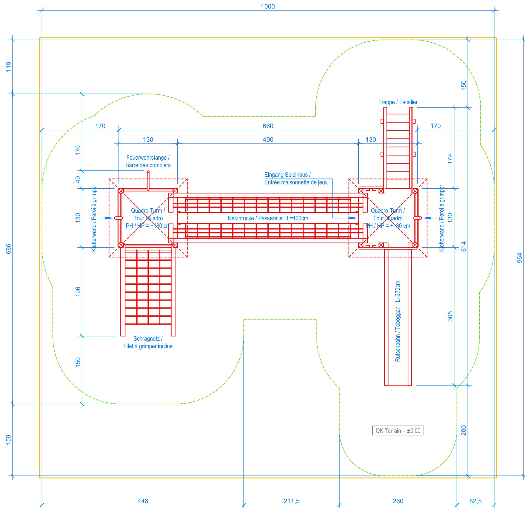
GRUNDRISS / PLAN 1:50
