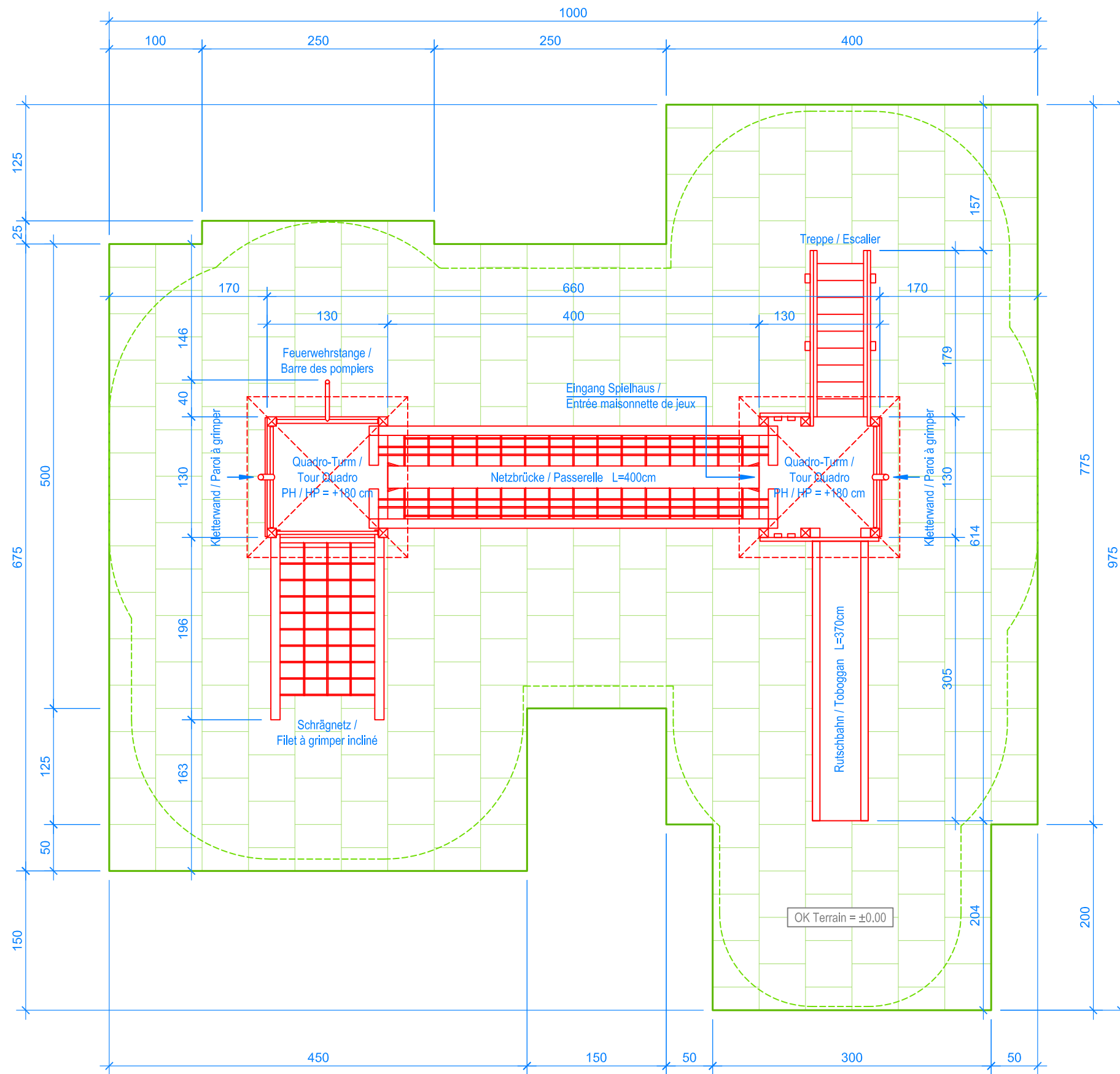
GRUNDRISS / PLAN 1:50
