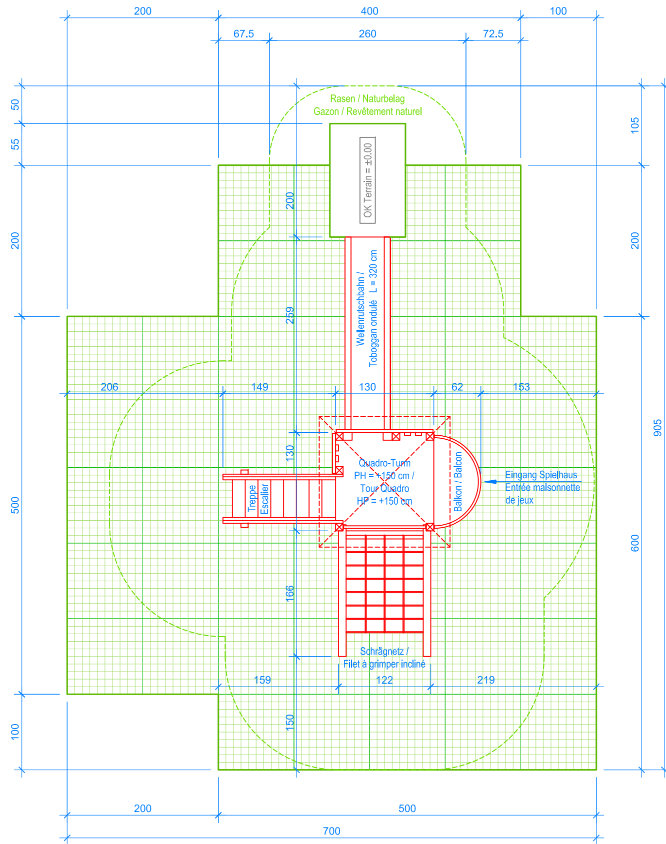
GRUNDRISS / PLAN 1:50
