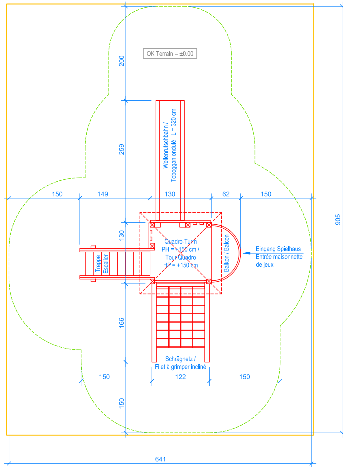
GRUNDRISS / PLAN 1:50
