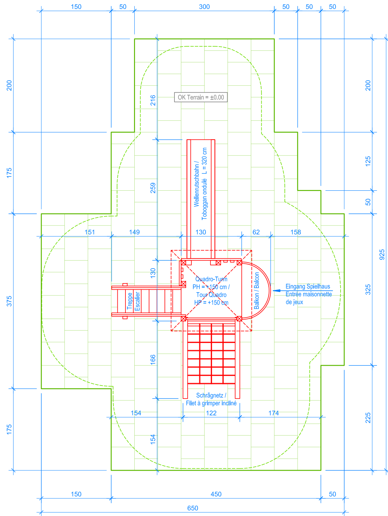
GRUNDRISS / PLAN 1:50
