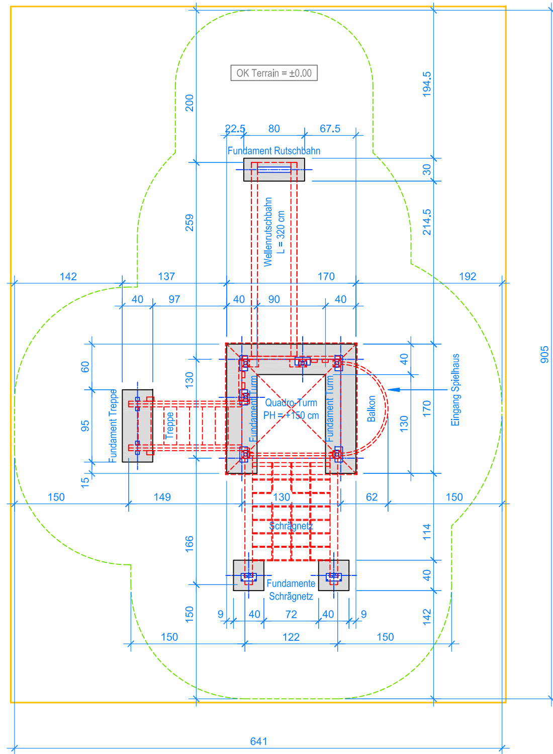
GRUNDRISS 1:50
