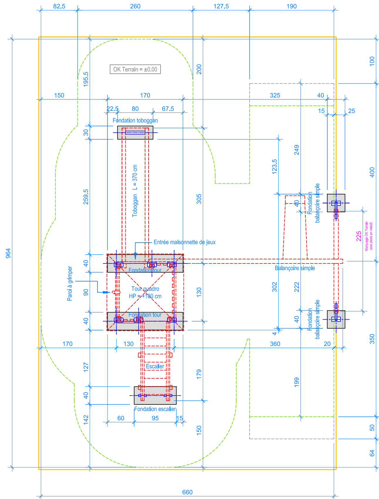
PLAN 1:50
