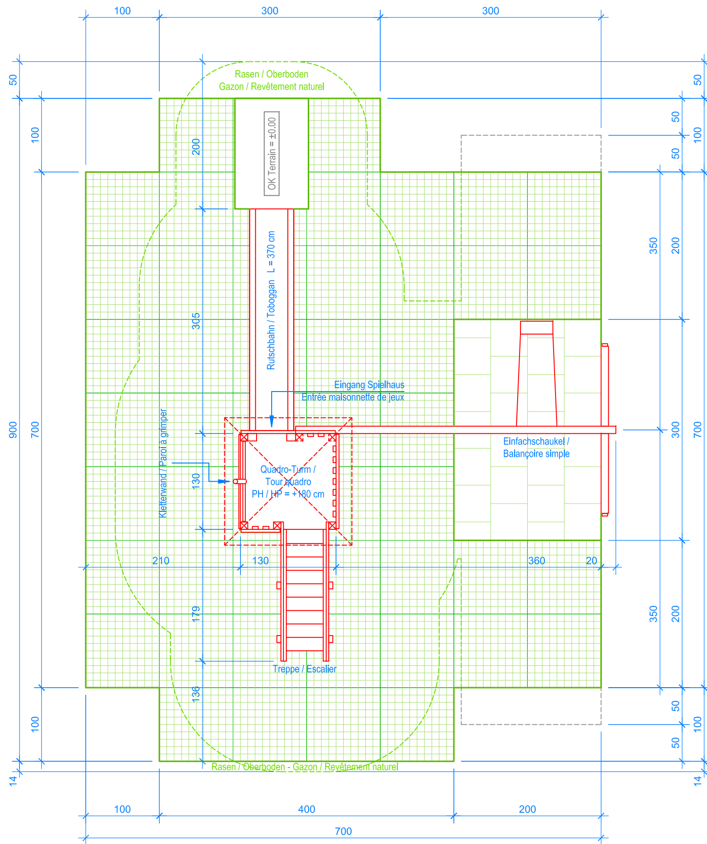
GRUNDRISS / PLAN 1:50
