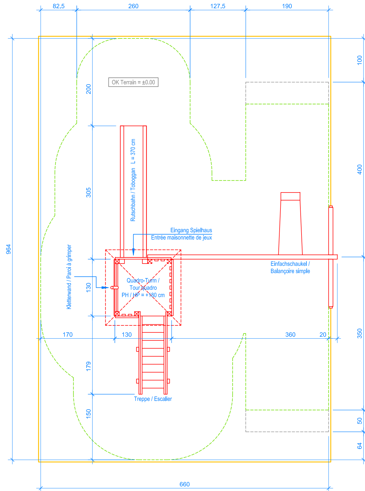
GRUNDRISS / PLAN 1:50
