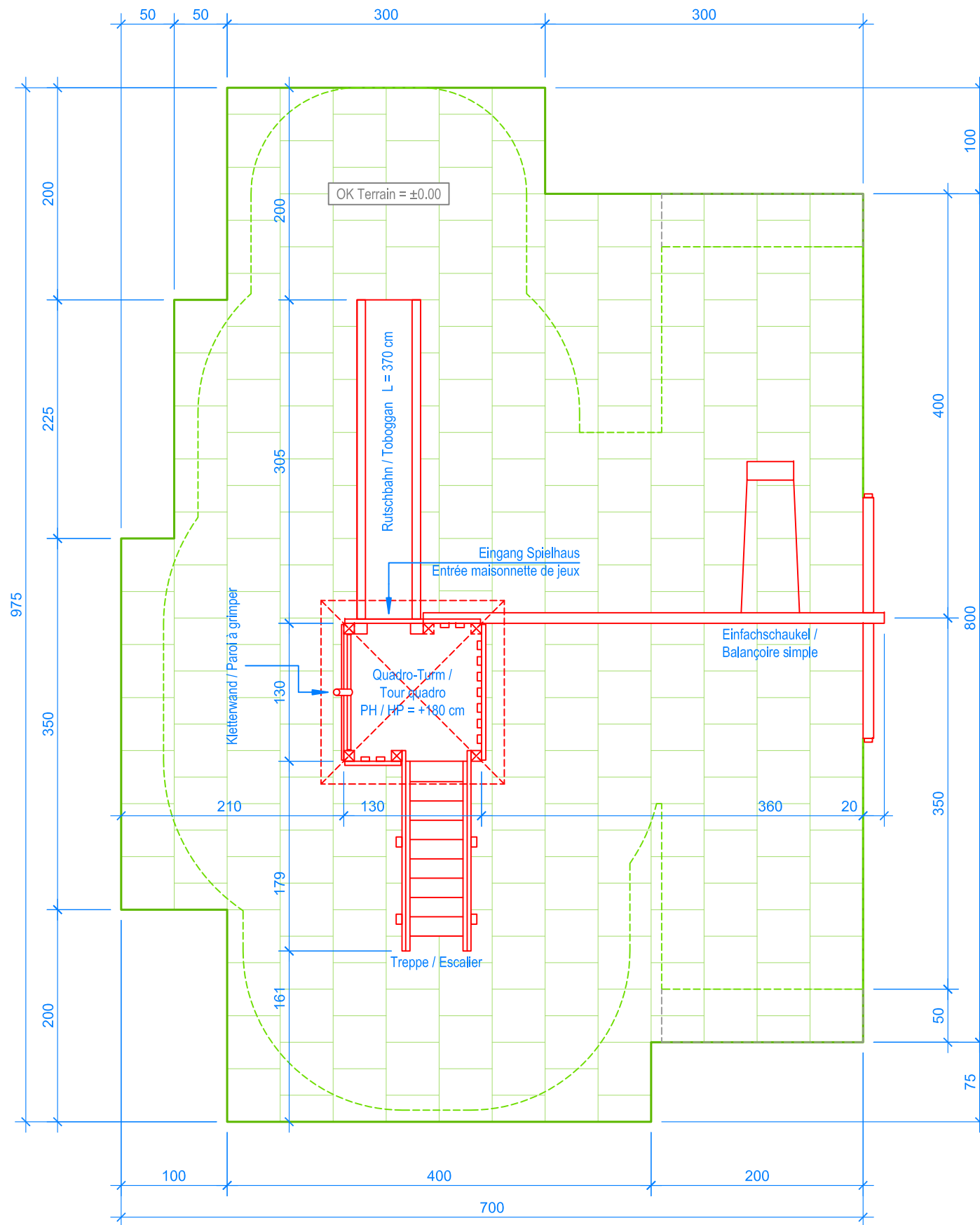
GRUNDRISS / PLAN 1:50
