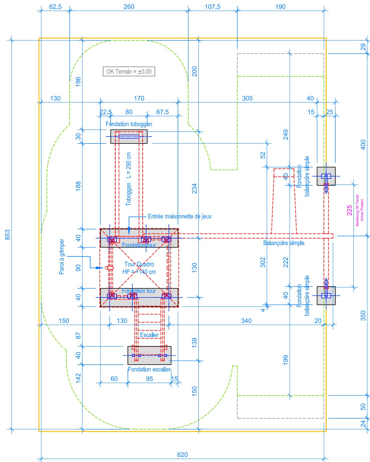
PLAN 1:50
