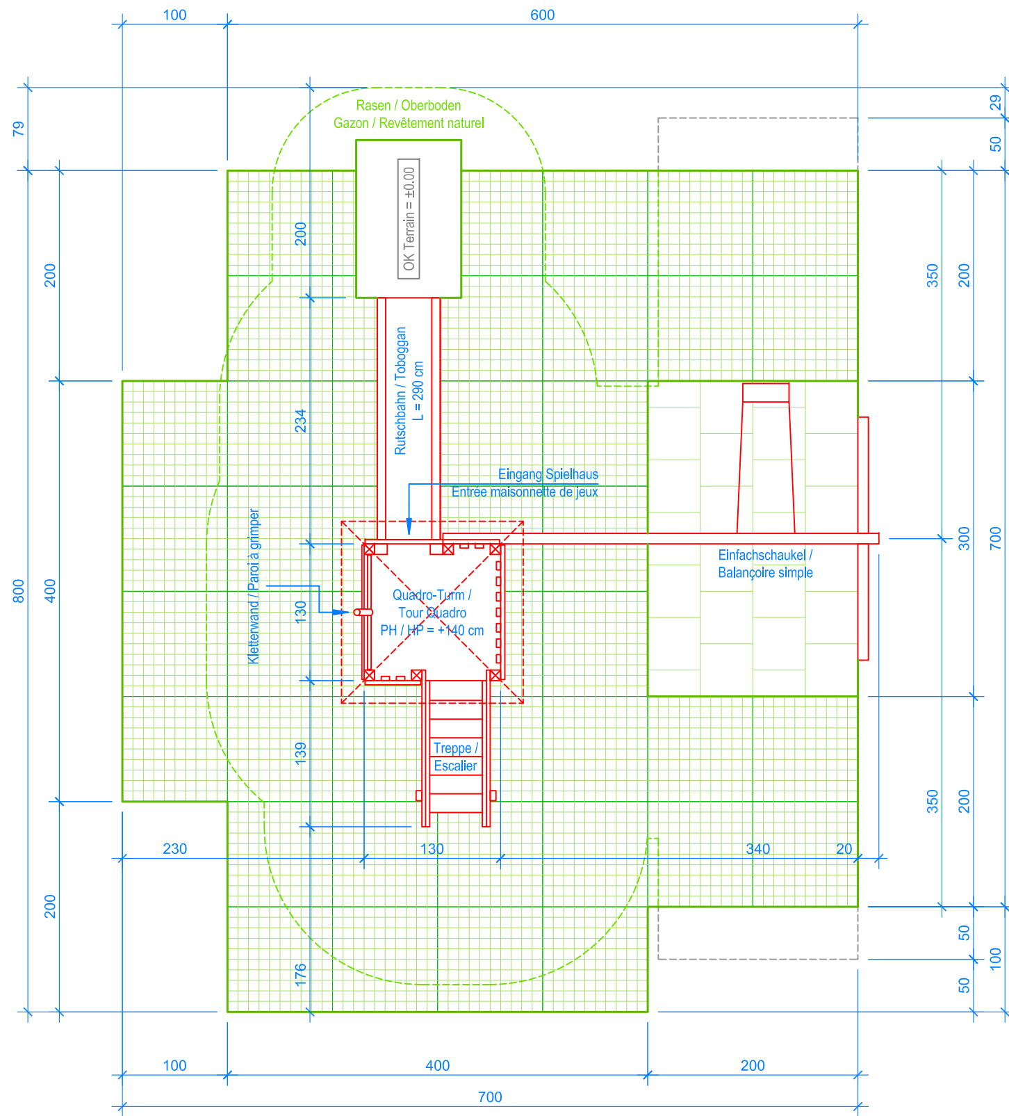
GRUNDRISS / PLAN 1:50
