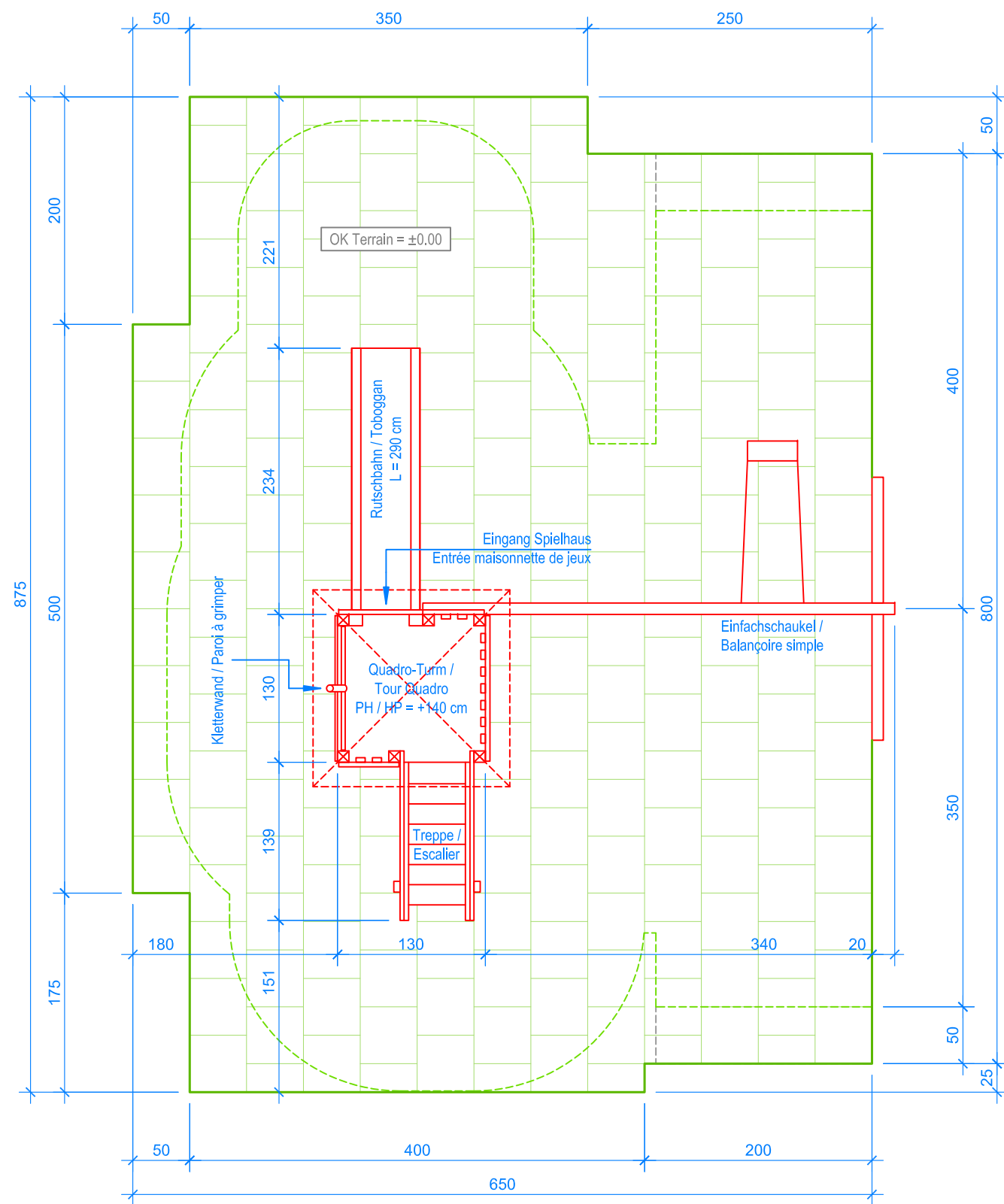
GRUNDRISS / PLAN 1:50
