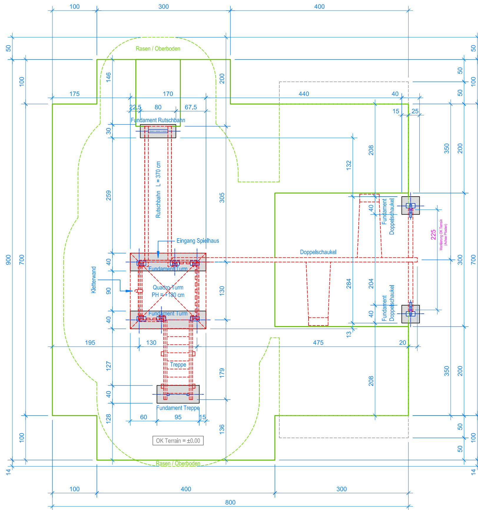
GRUNDRISS 1:50
