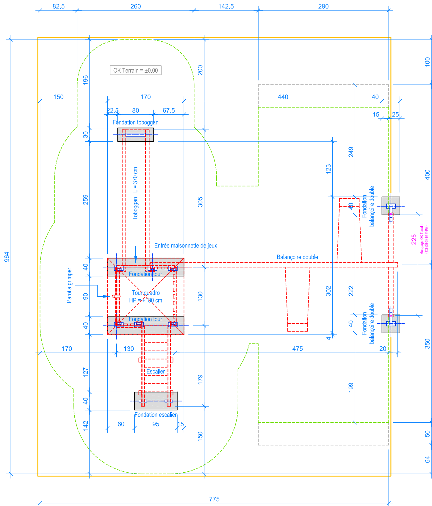
PLAN 1:50
