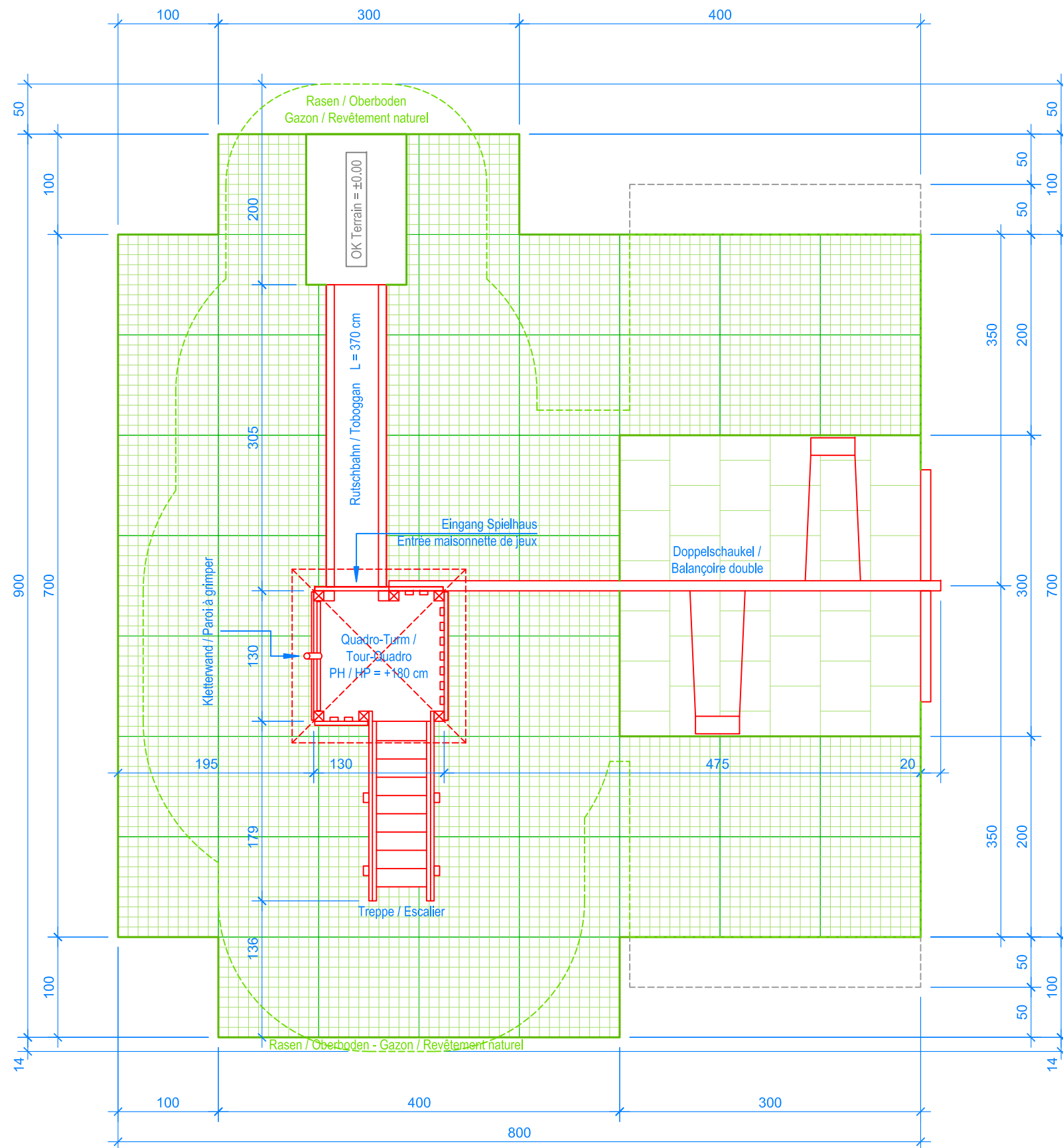
GRUNDRISS / PLAN 1:50
