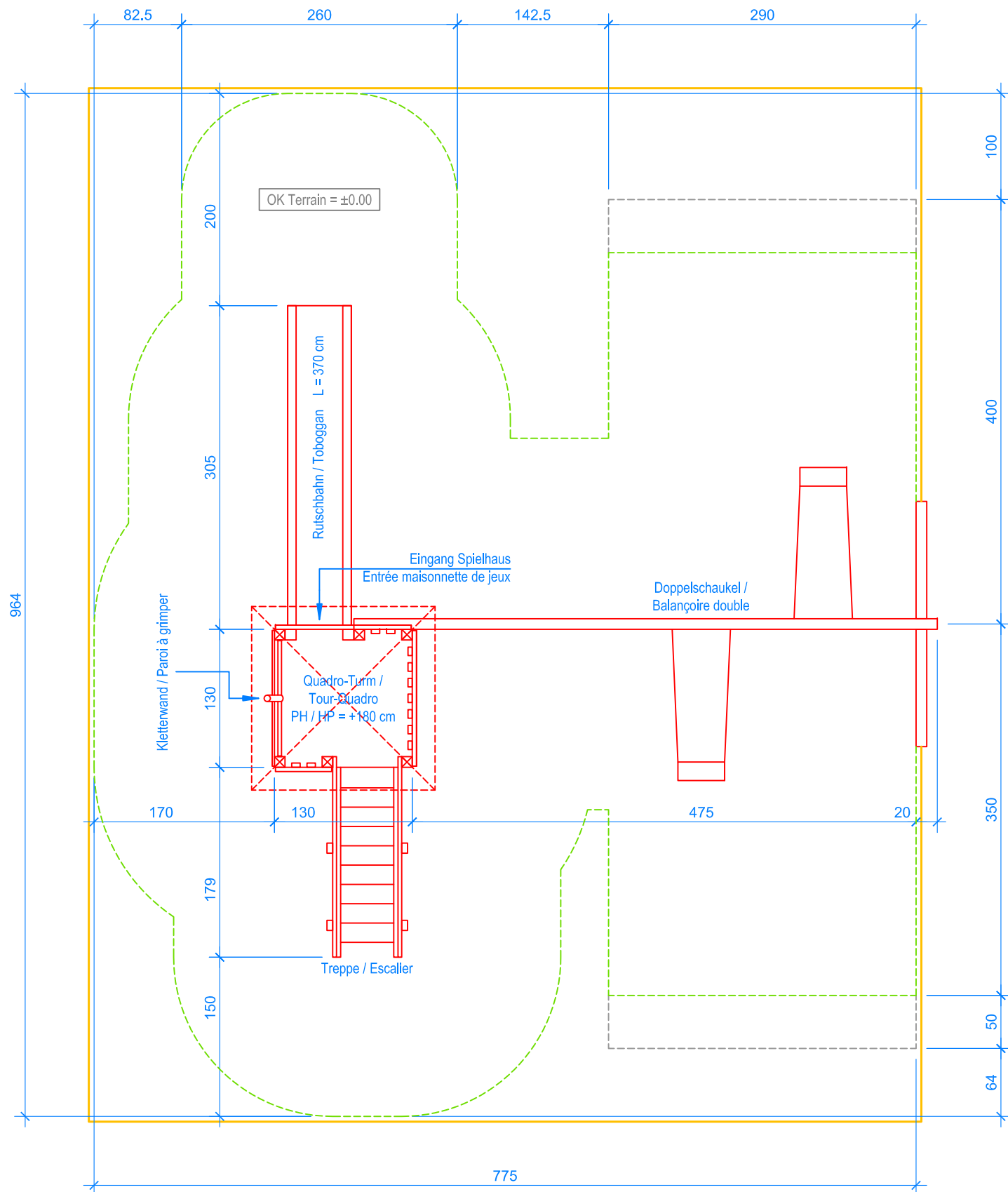
GRUNDRISS / PLAN 1:50
