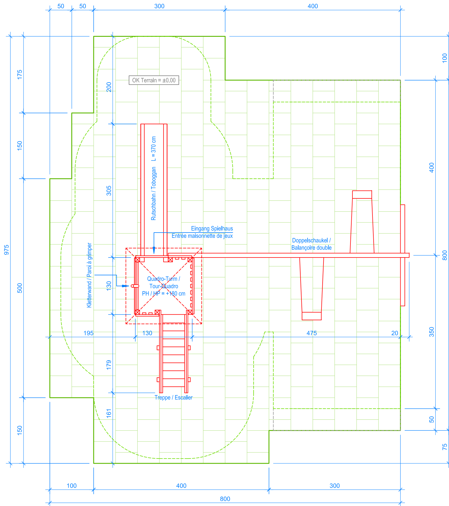
GRUNDRISS / PLAN 1:50
