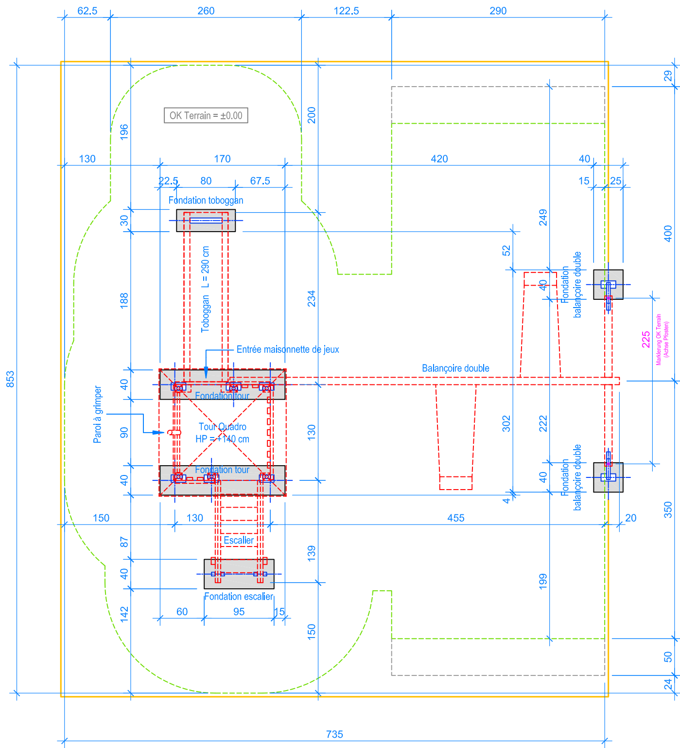
PLAN 1:50
