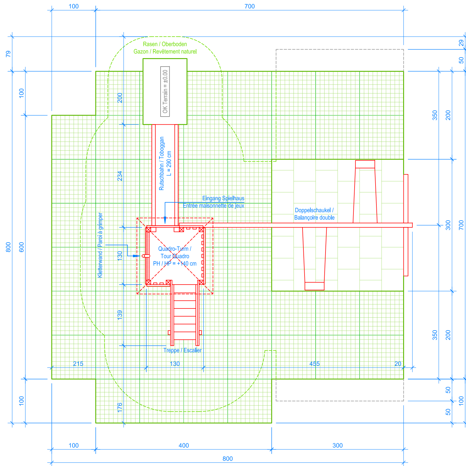
GRUNDRISS / PLAN 1:50
