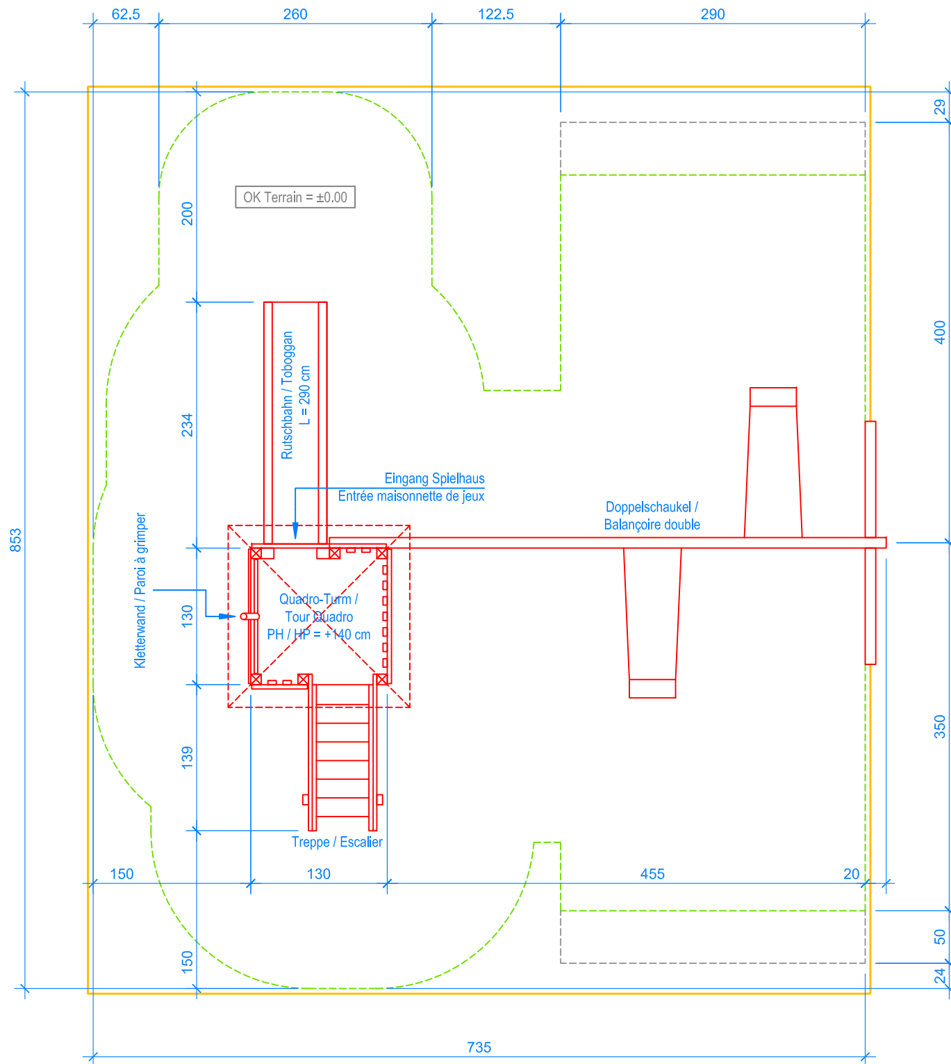
GRUNDRISS / PLAN 1:50
