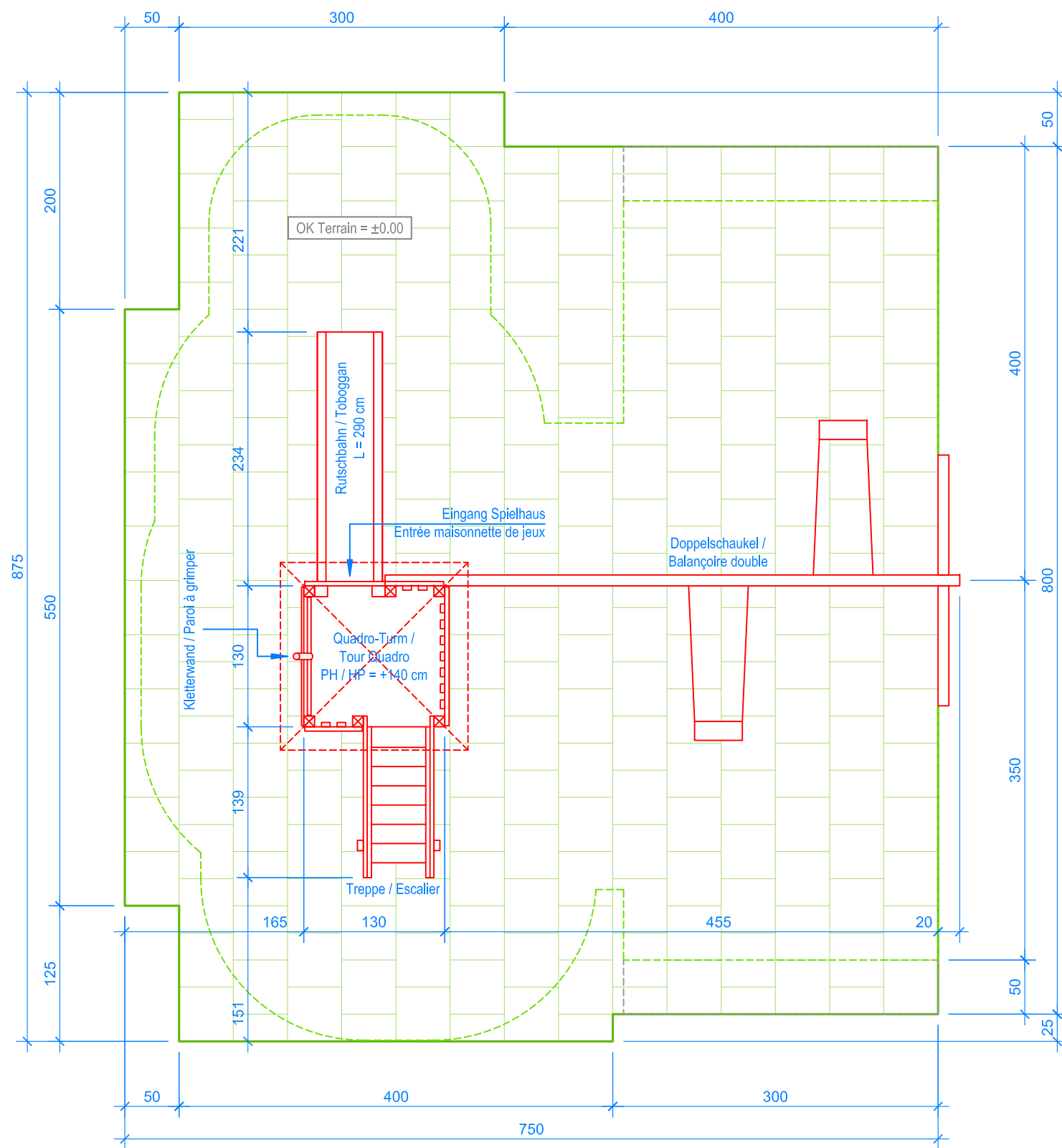
GRUNDRISS / PLAN 1:50
