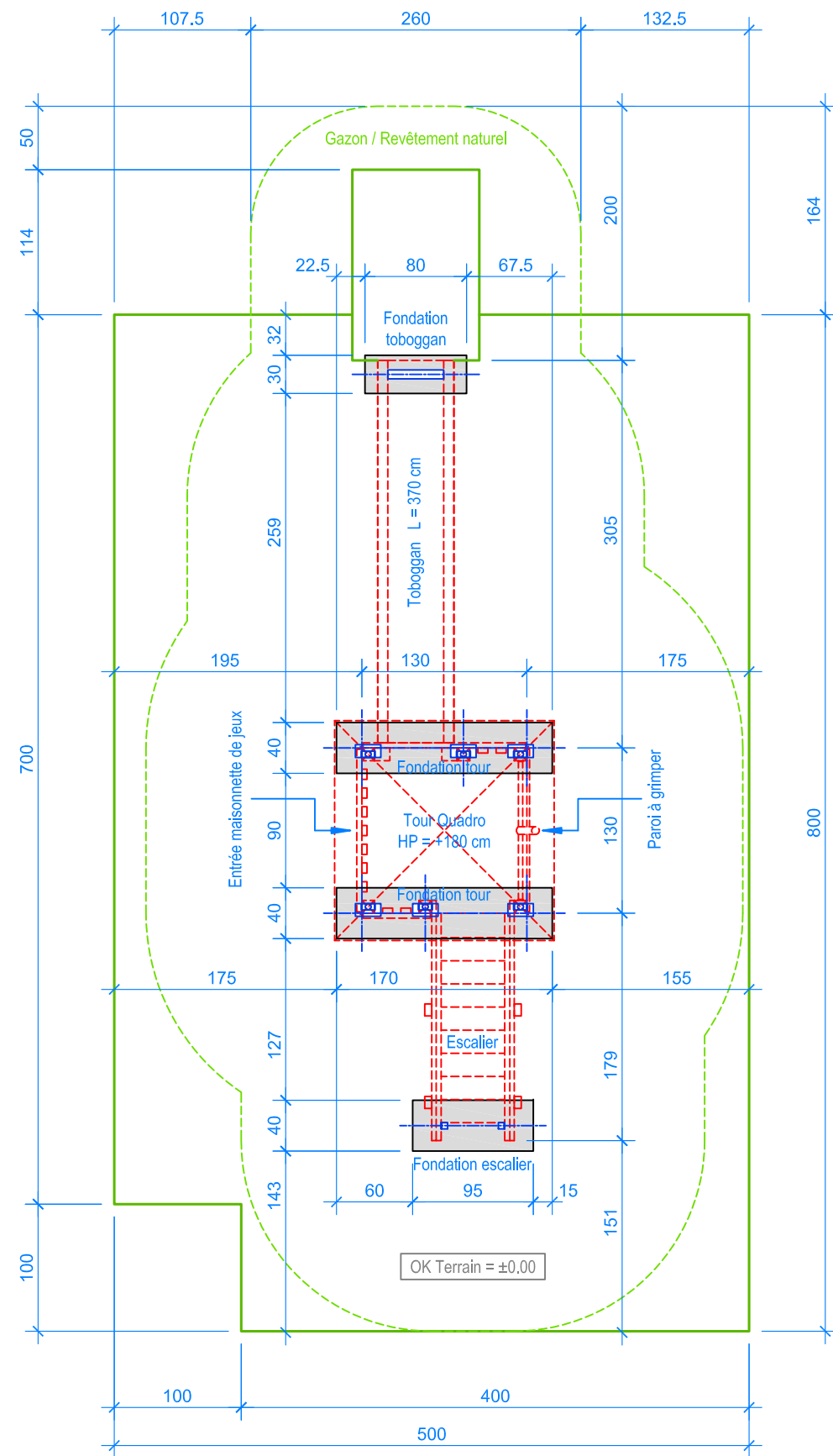
PLAN 1:50
