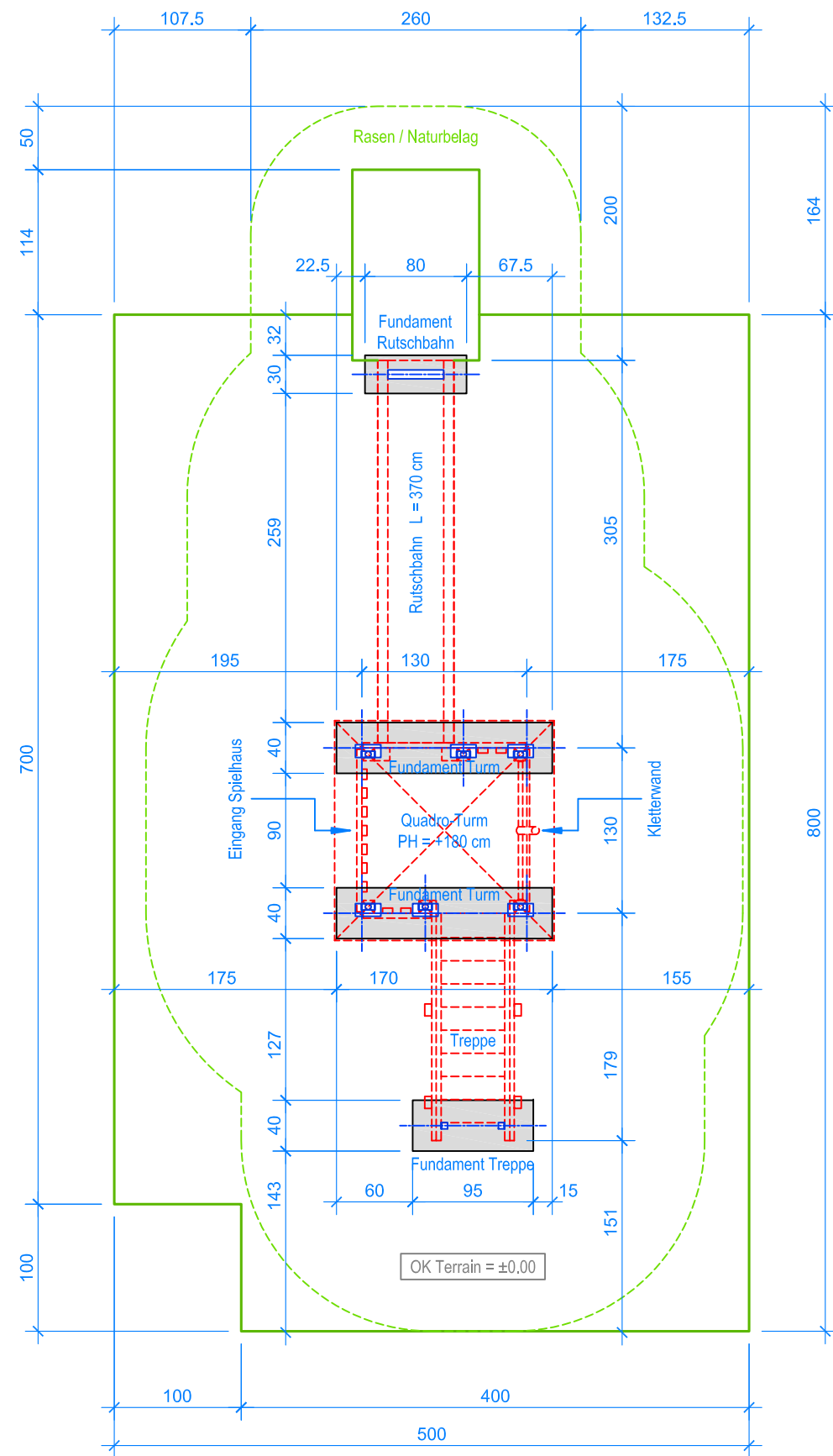
GRUNDRISS 1:50
