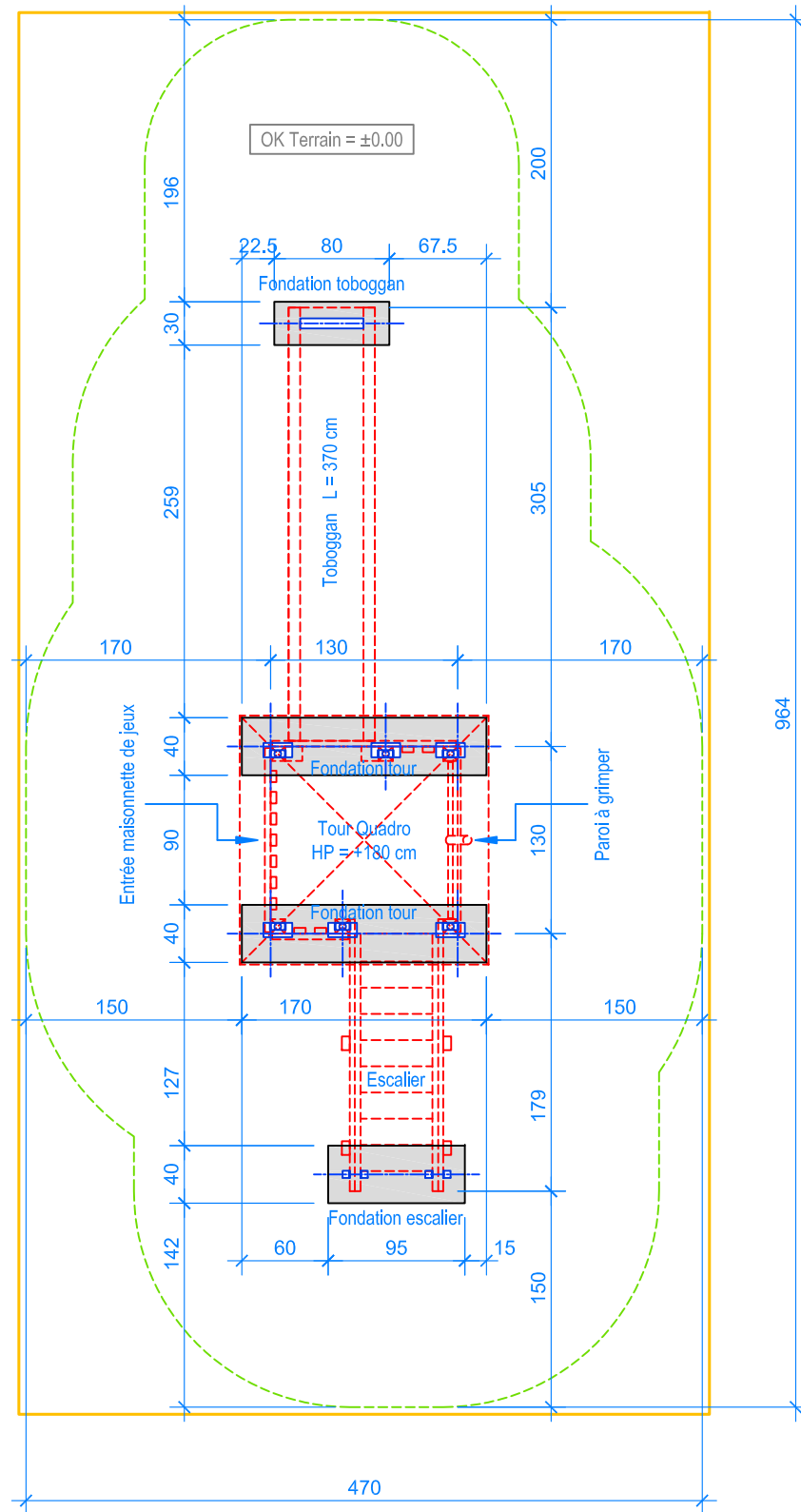
PLAN 1:50
