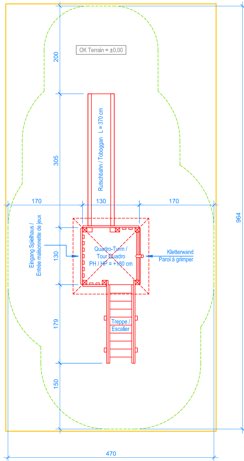
GRUNDRISS / PLAN 1:50
