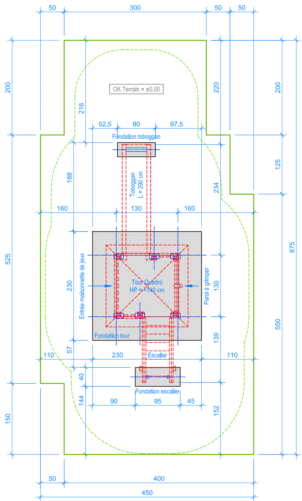
PLAN 1:50
