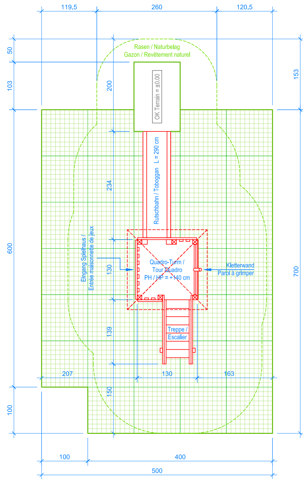
GRUNDRISS / PLAN 1:50
