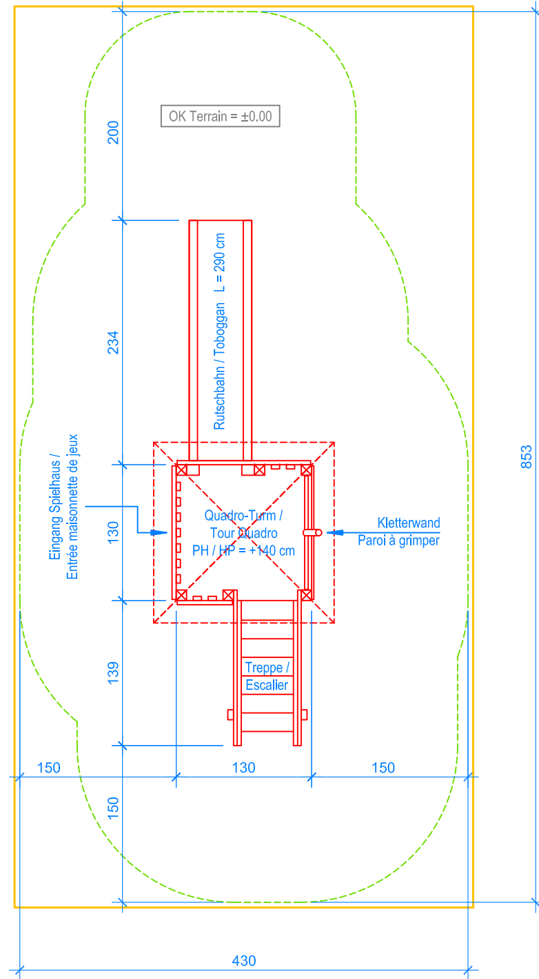
GRUNDRISS / PLAN 1:50
