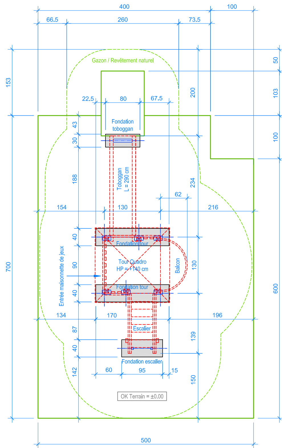
PLAN 1:50
