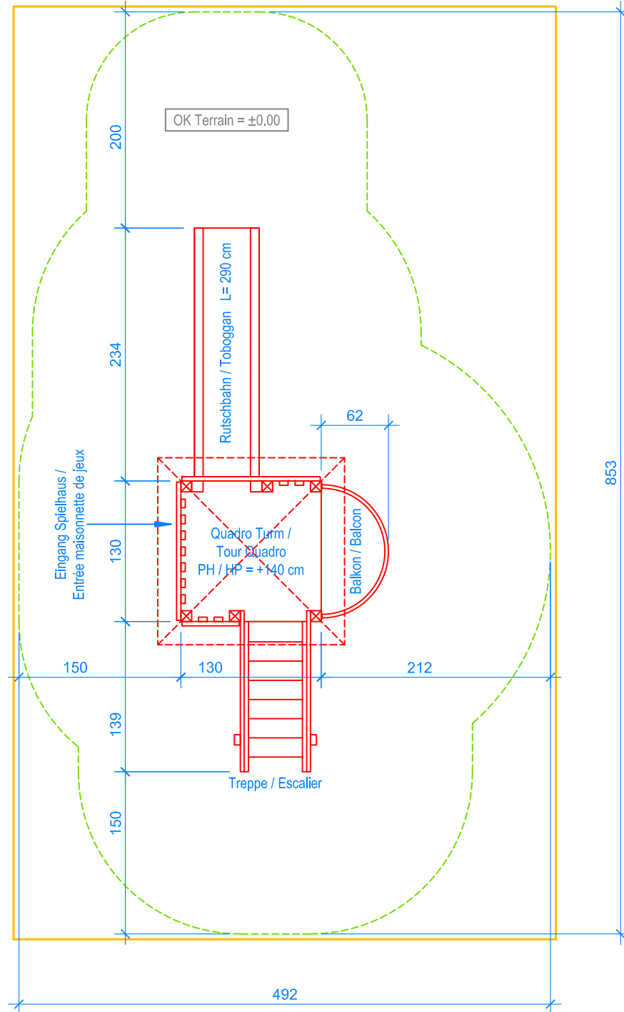
GRUNDRISS / PLAN 1:50
