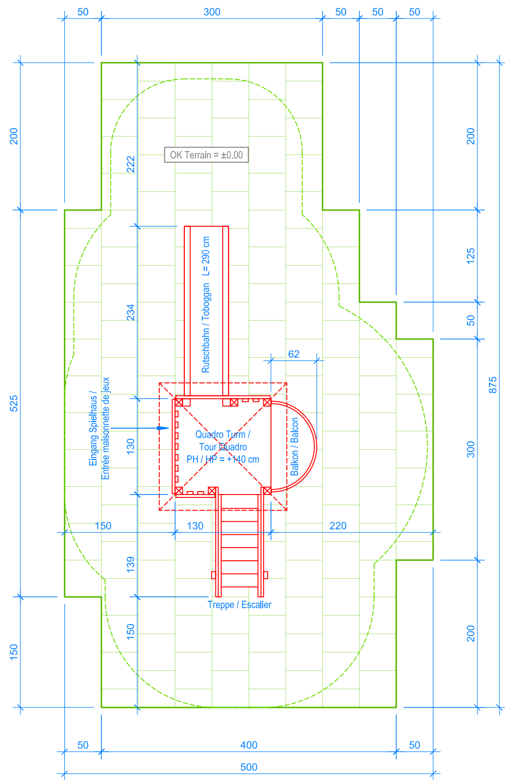
GRUNDRISS / PLAN 1:50
