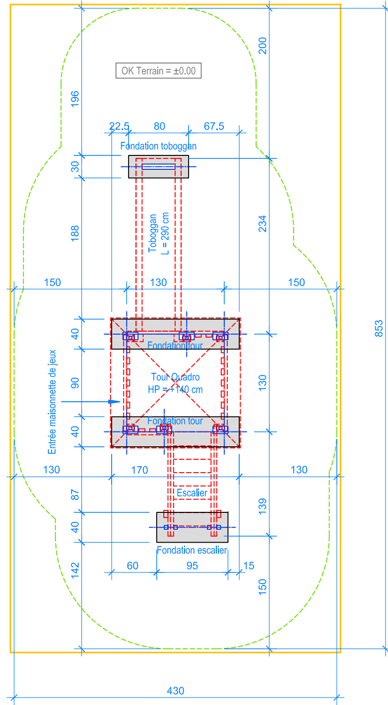
PLAN 1:50
