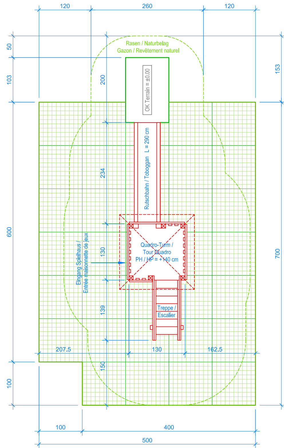
GRUNDRISS / PLAN 1:50
