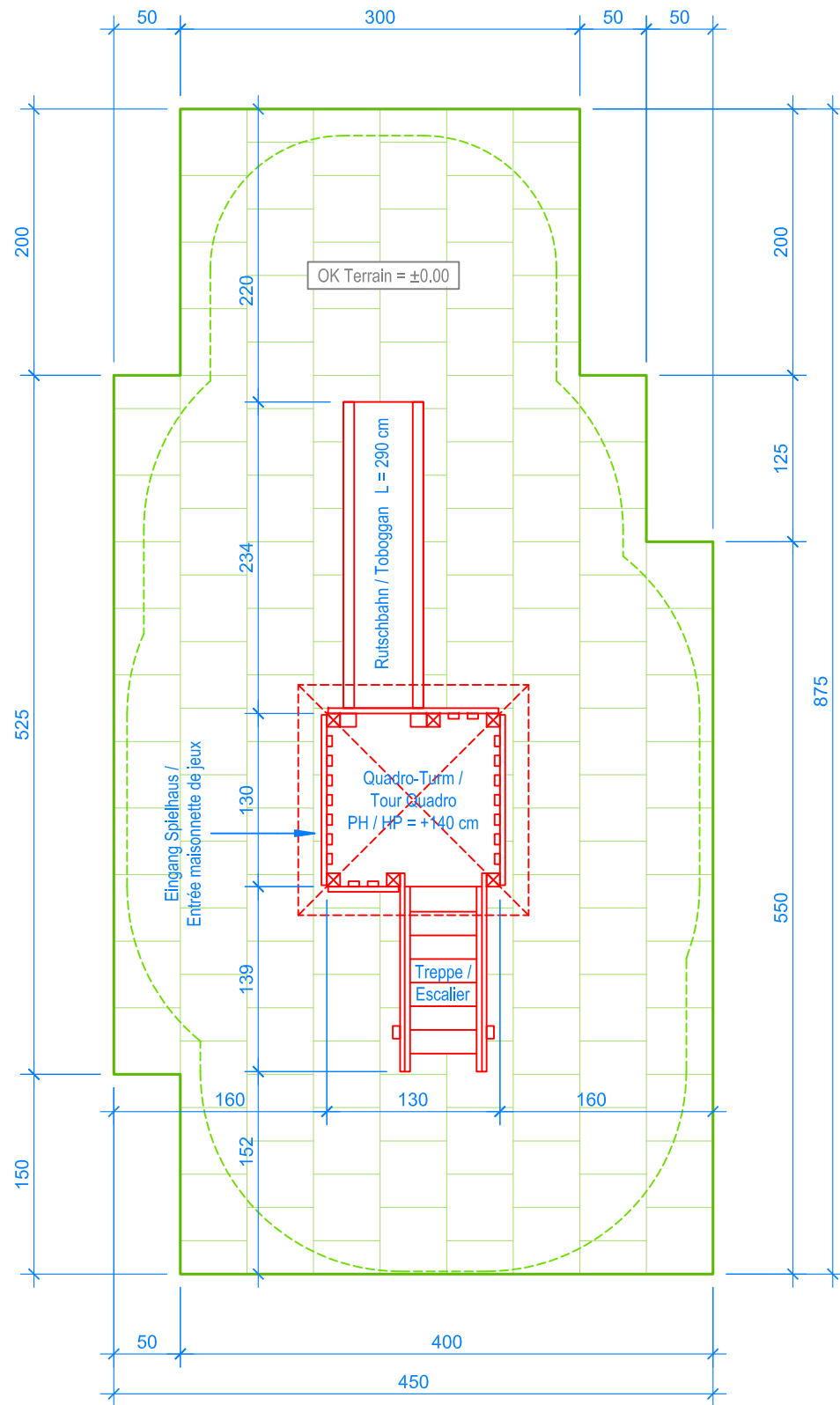
GRUNDRISS / PLAN 1:50
