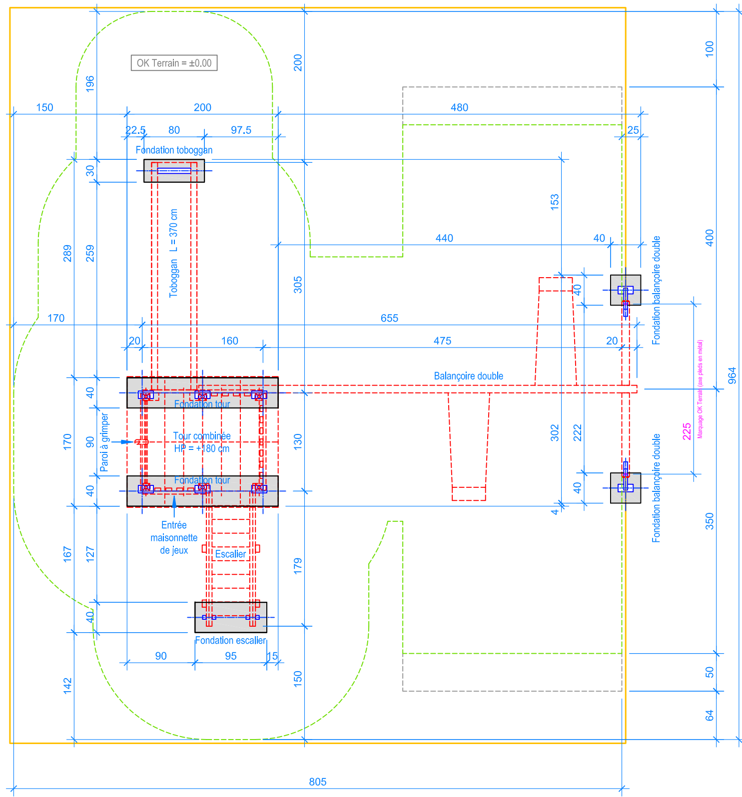
PLAN 1:50
