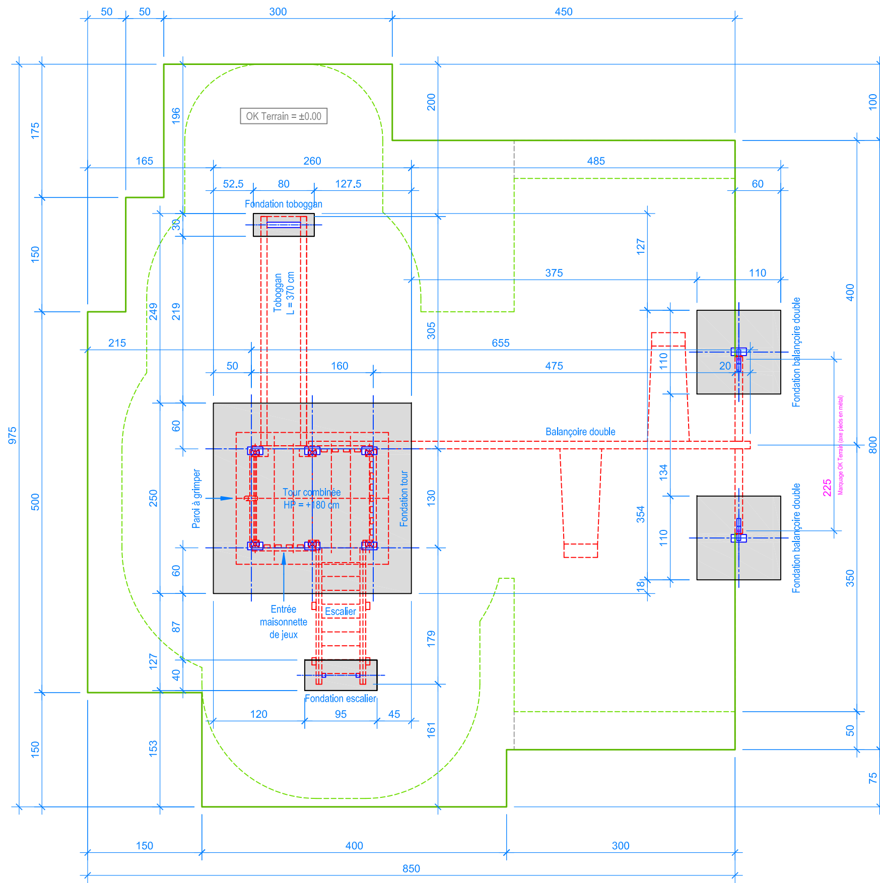
PLAN 1:50
