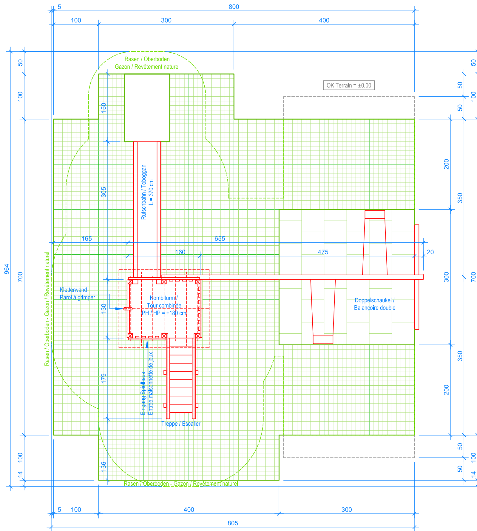
GRUNDRISS / PLAN 1:50
