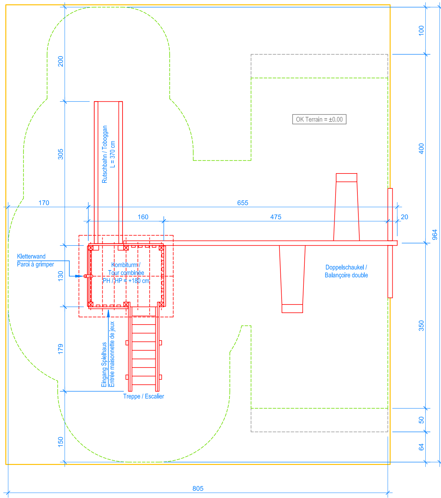
GRUNDRISS / PLAN 1:50
