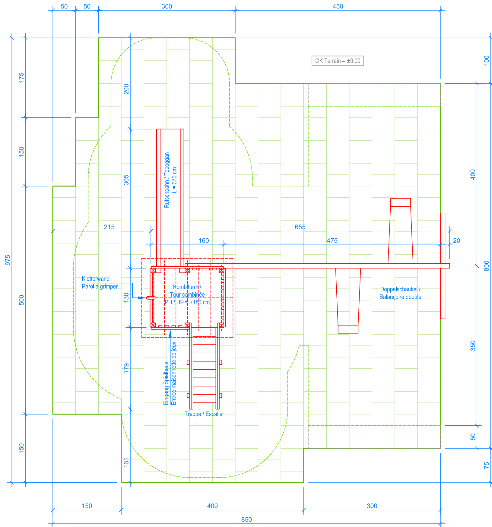
GRUNDRISS / PLAN 1:50
