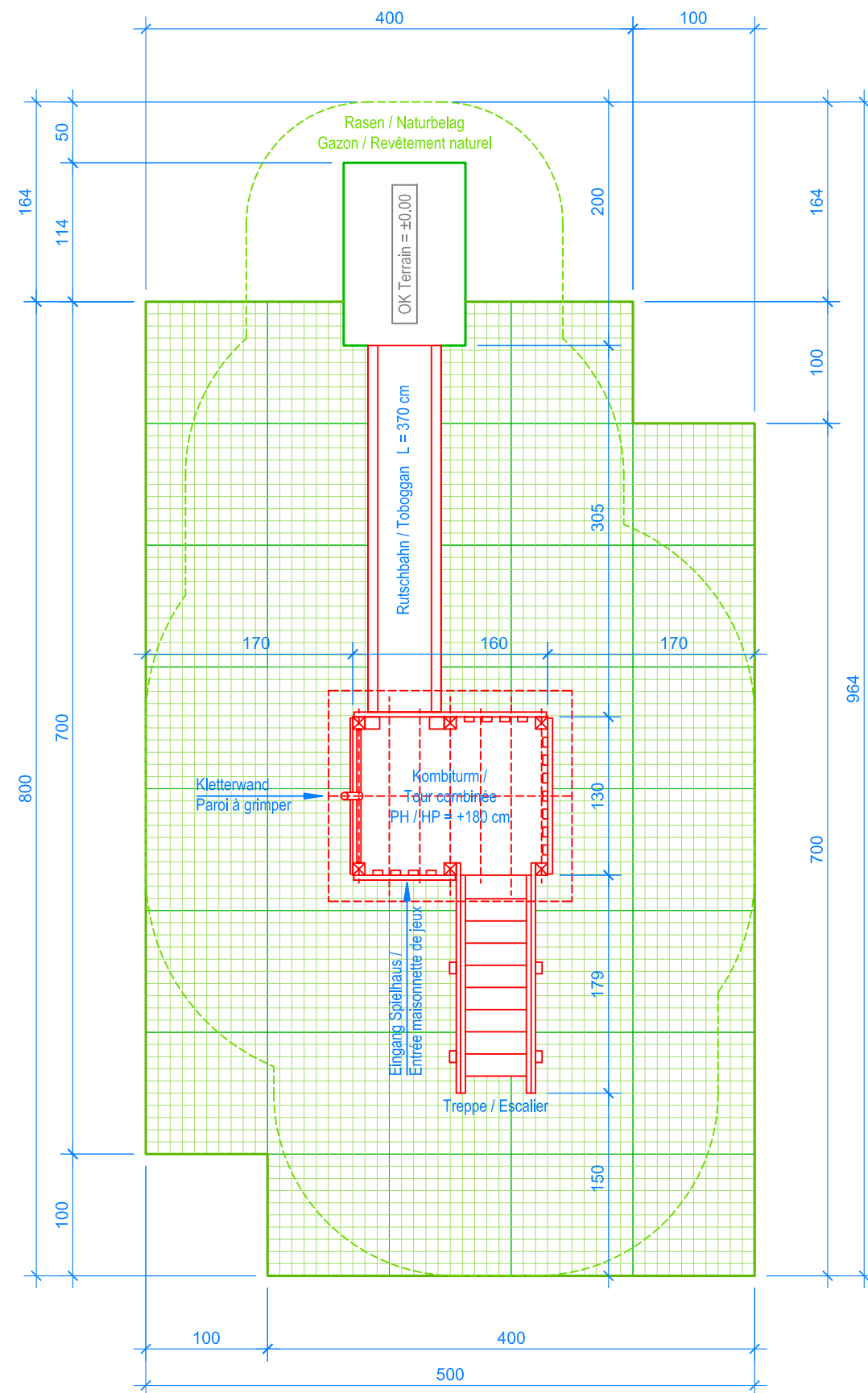
GRUNDRISS / PLAN 1:50
