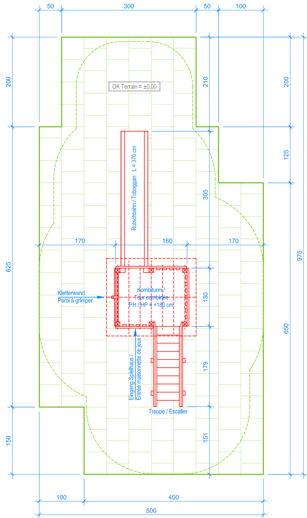
GRUNDRISS / PLAN 1:50
