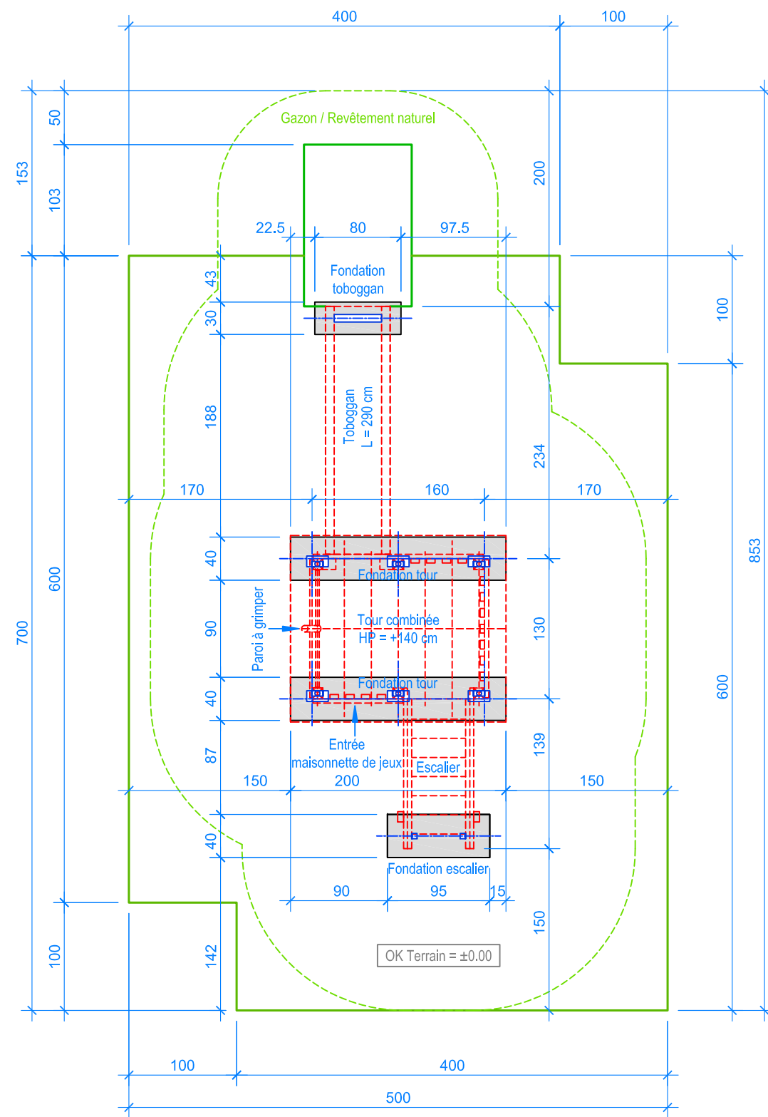
PLAN 1:50
