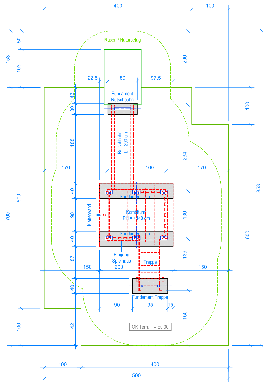
GRUNDRISS 1:50
