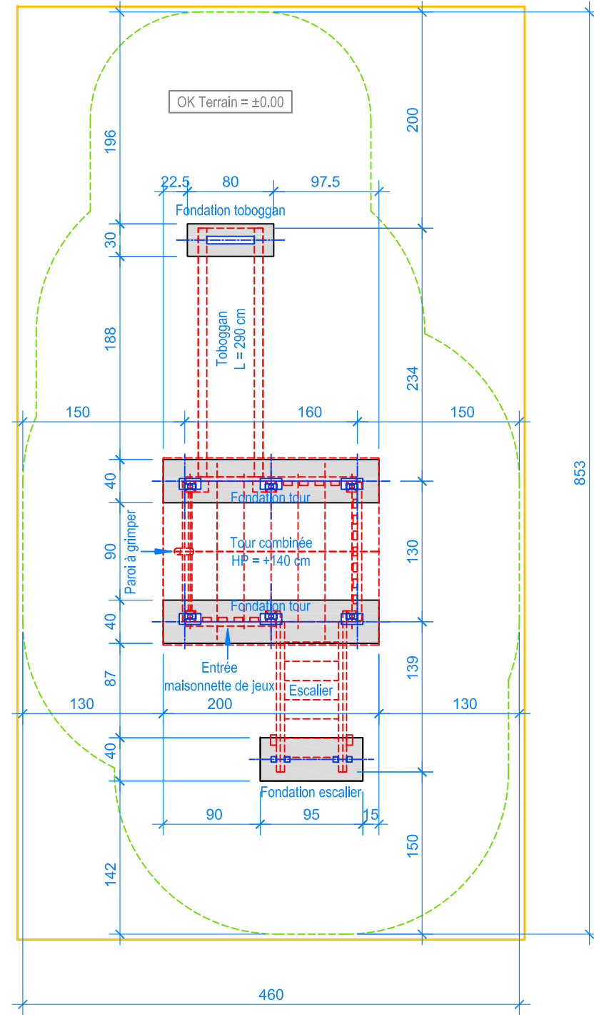
PLAN 1:50
