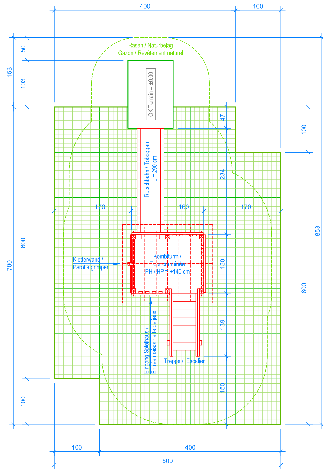
GRUNDRISS / PLAN 1:50
